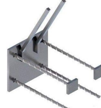
Закладные MN301-MN305
