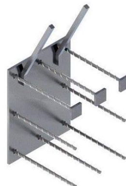
Закладные MN312-MN313
