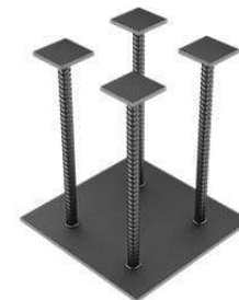
Закладные МН105-МН116
