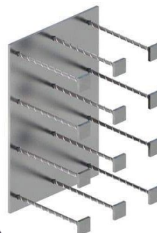
Закладные МН163-МН164
