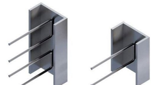
Закладные МН558-МН565
